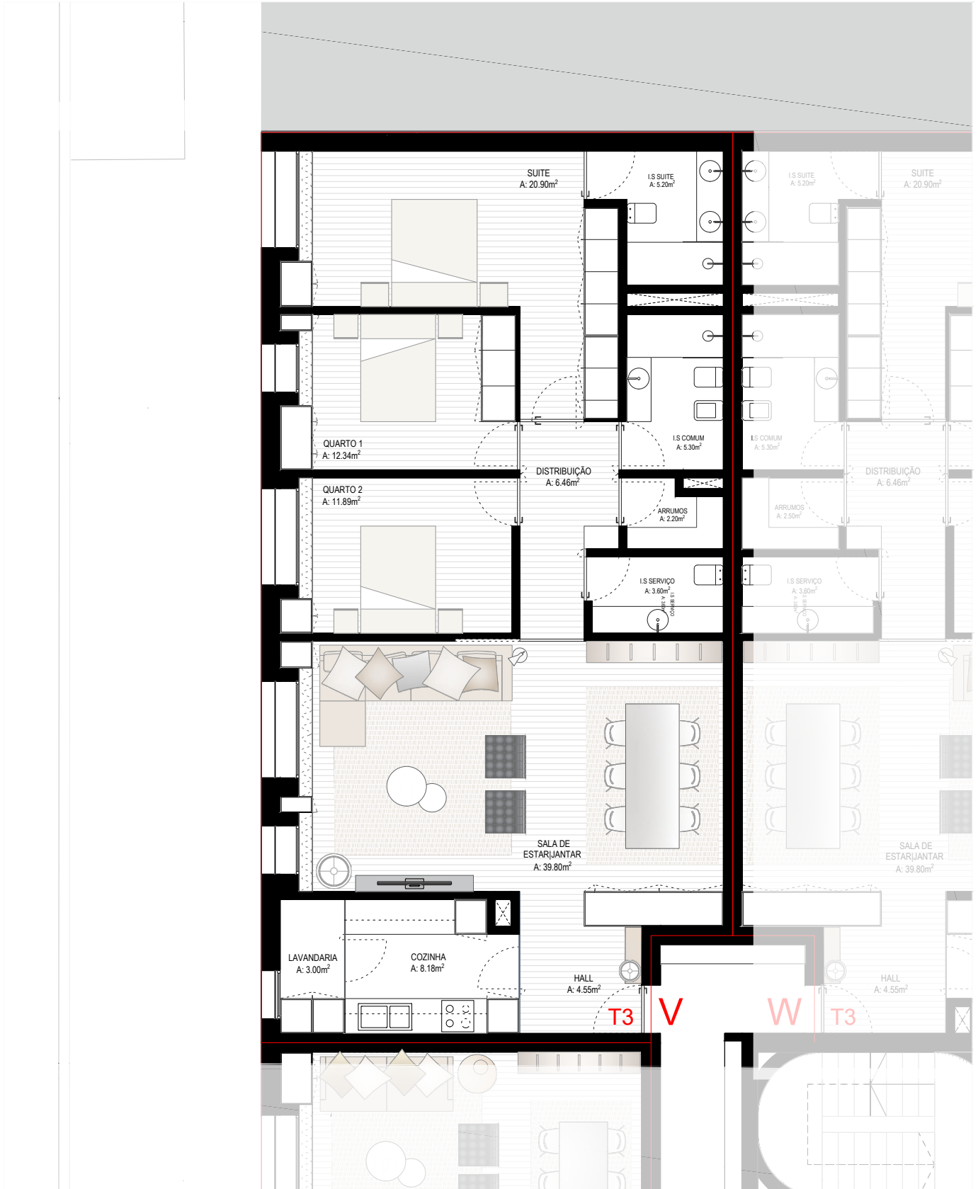
Planta Piso 3 escala 1:100
