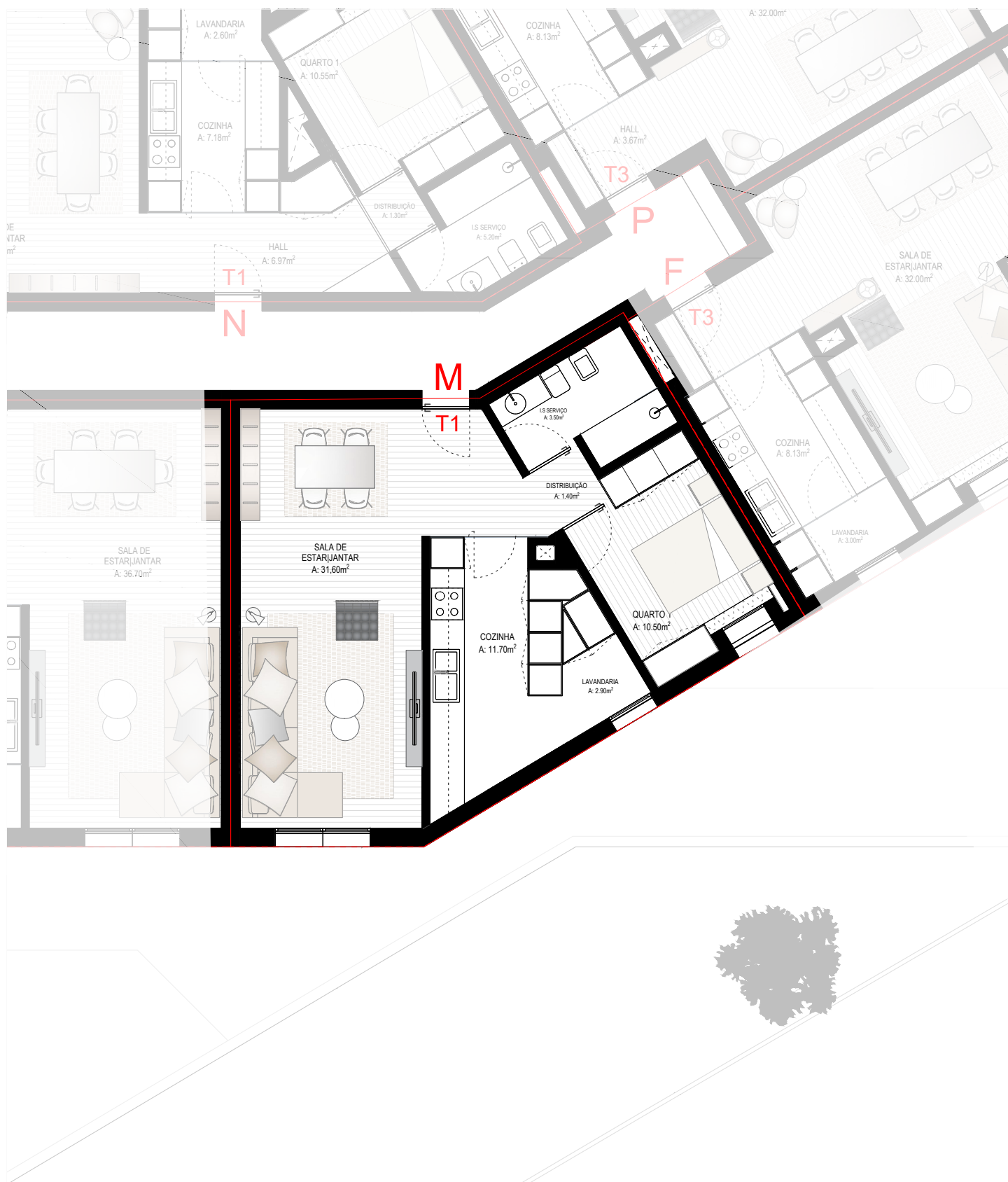
Planta Piso 1 escala 1:100
